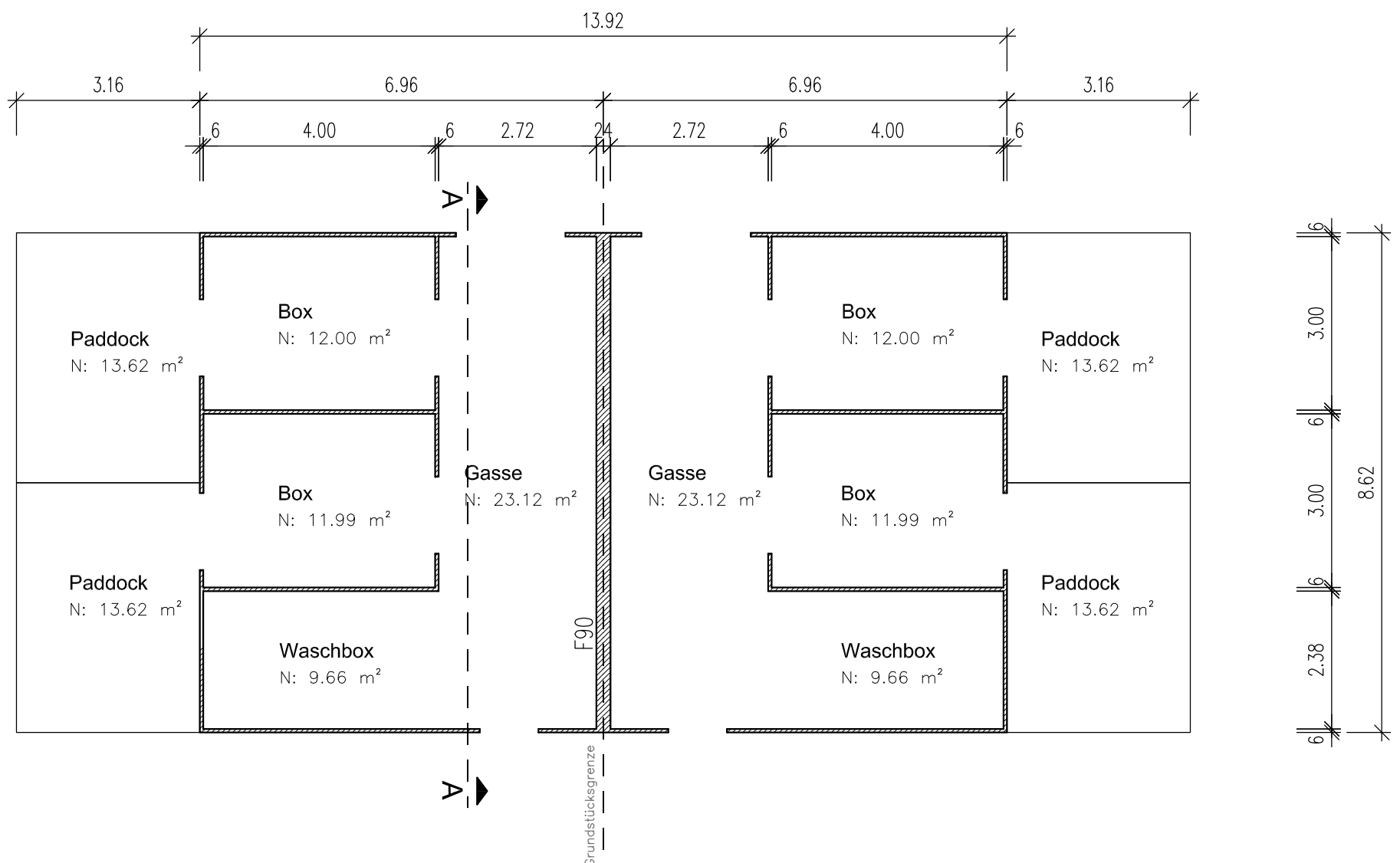
Grundriss
